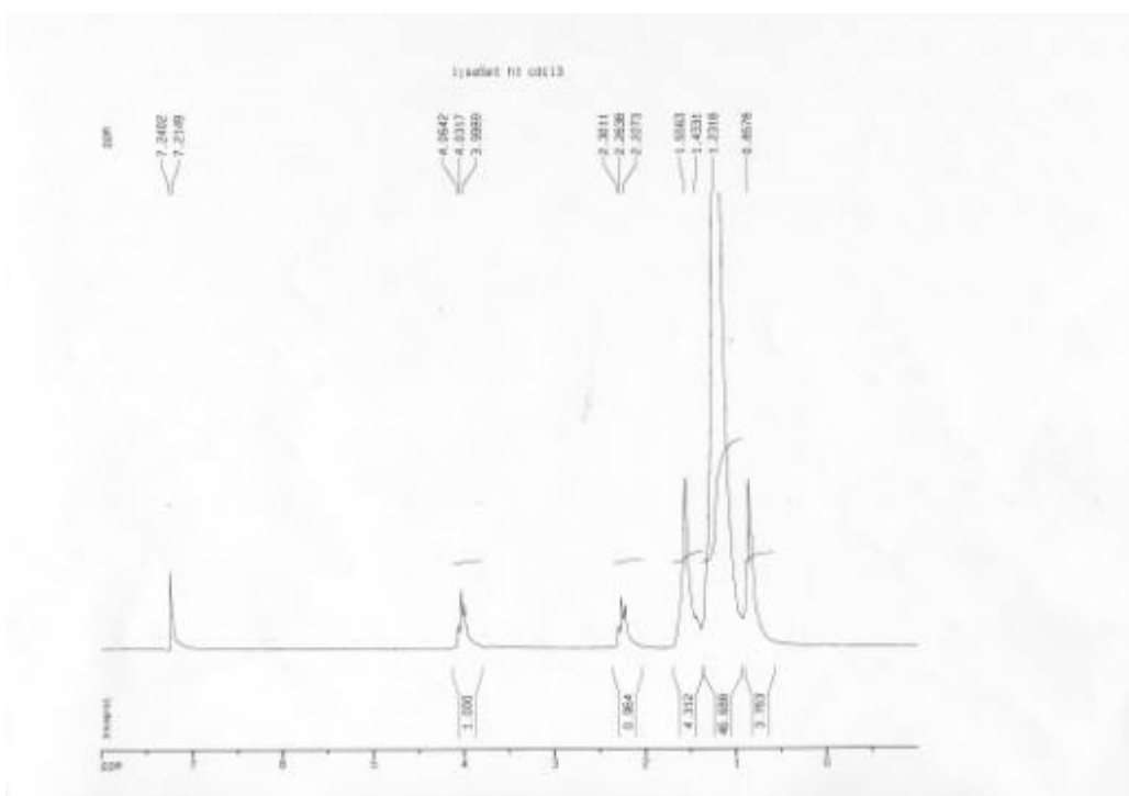
圖 8 : ^1\text{H} -NMR spectrum of compound III
