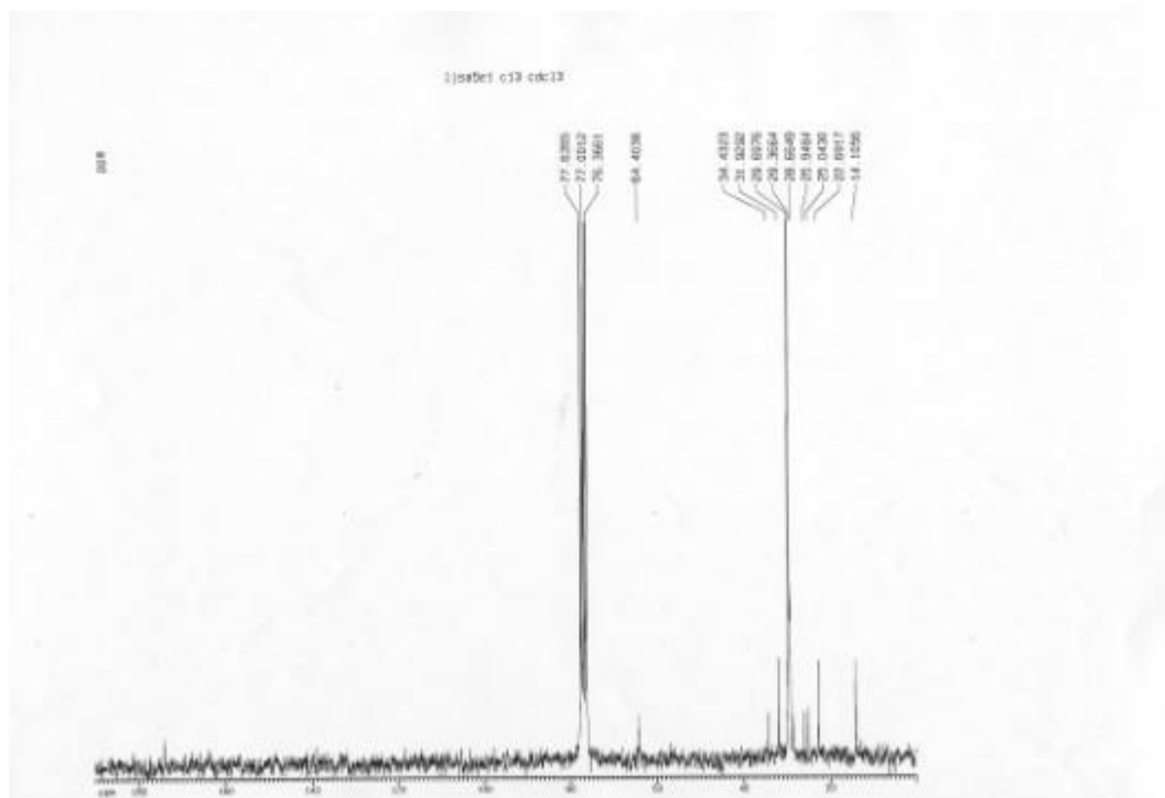
圖 9 : ^{13}\text{C} -NMR spectrum of compound III
